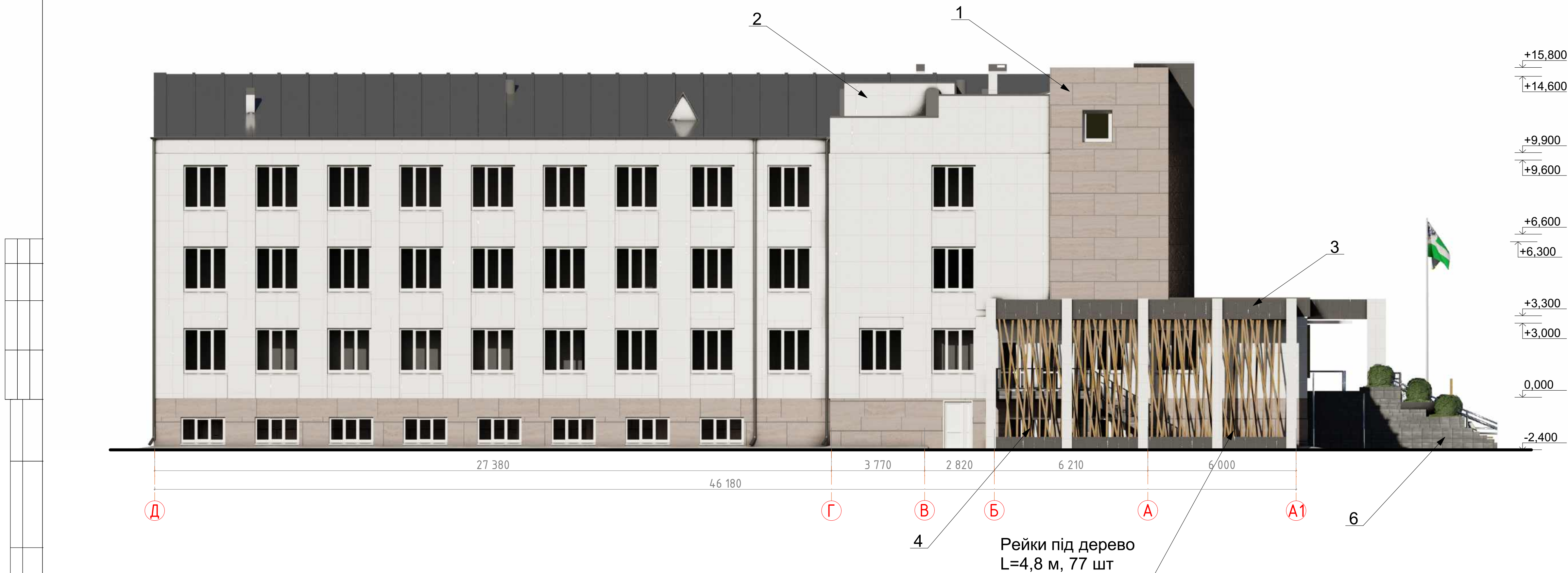
Фасад Д-А1 М 1:100
